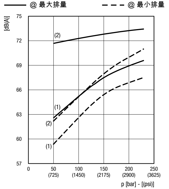
噪音水平 麦克风到泵的距离 = 1 m (39.37 in)
