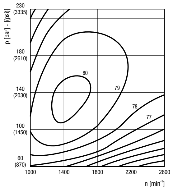
整体效率 @最大排量
