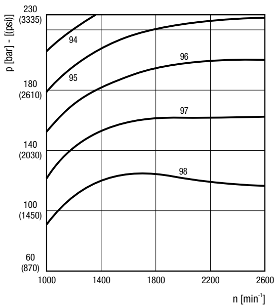
容积效率 @最大排量
