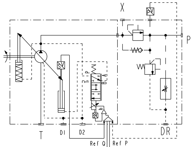
DESR 液压回路
